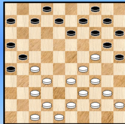
14-19 ?
