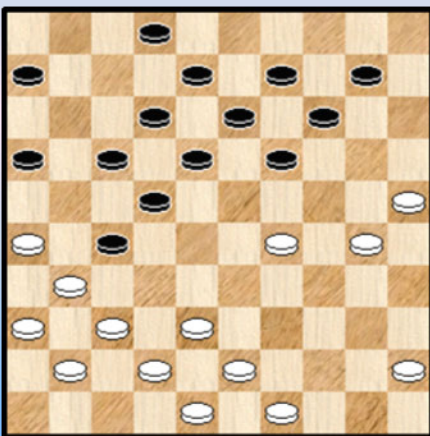
19-23 ?
