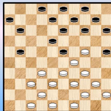
33-28 ?
