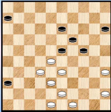
Diagram 8A Waz
