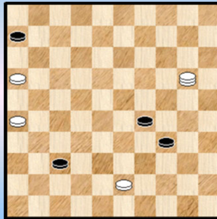
Diagram 5 Eindstand
