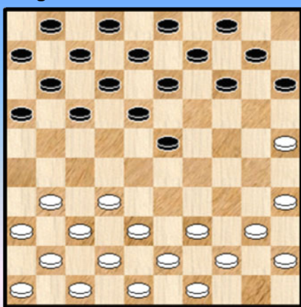
Diagram 3 Zaz
