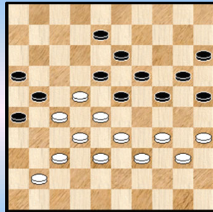
24-30 ?
