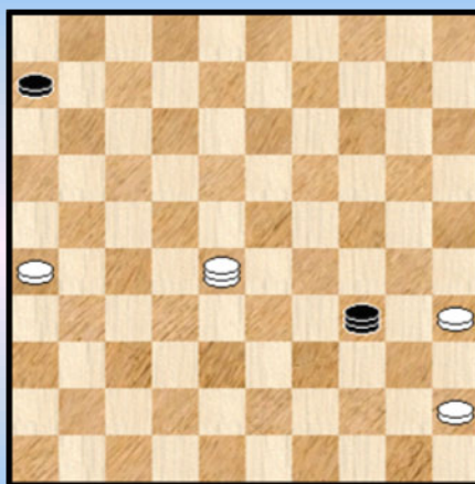
Diagram 8B 26-21 ?
