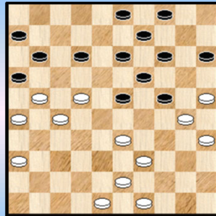
48-42 ?
