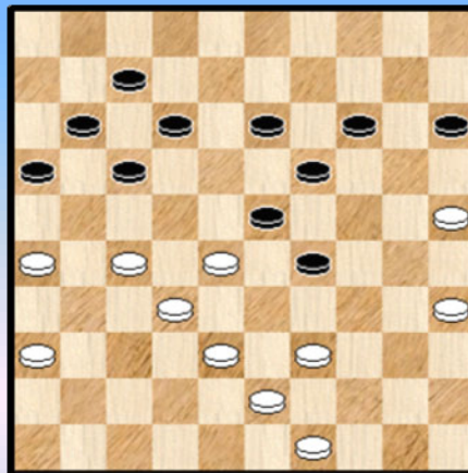
Diagram 6 49-44 ?
