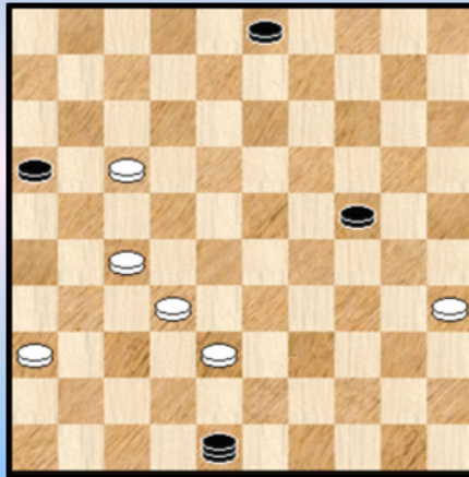
Diagram 2A 48-26 ?
