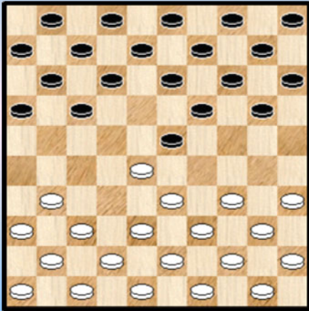
Diagram 1 37-32 ? 20-25 ?
