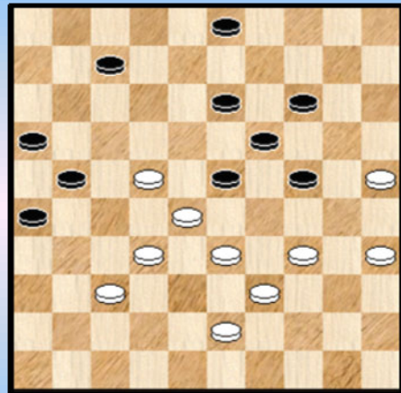
34-29 ?
