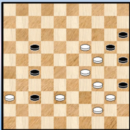
Diagram 18 Zaz
