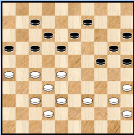
Andy Damen 28-23 ?
