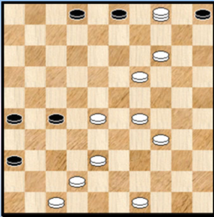
Diagram 43A 02-08 ?
