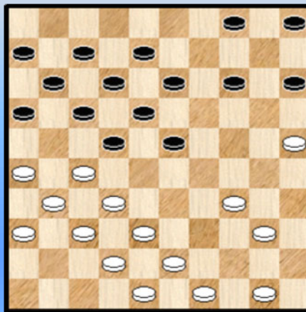
Diagram 2 49-44 ?
