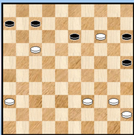
Diagram 8A Zaz
