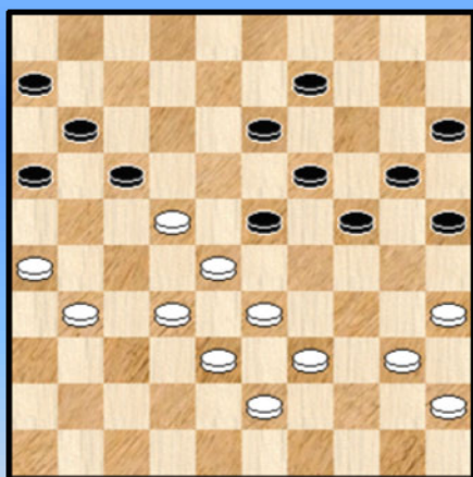
Diagram 19 25-30 ?
