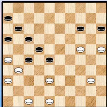
Diagram 3I 40-34 ?
