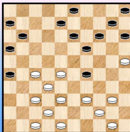
Diagram 21 03-09 ?
